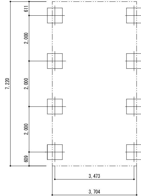
■ 基礎配置図
